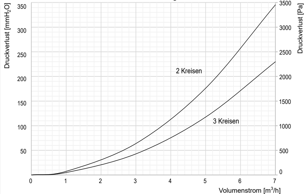
Druckverlustdiagramm
